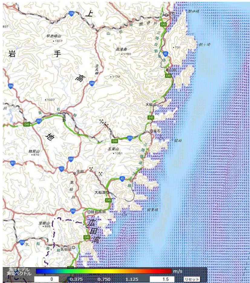
令和7年7月8日10時00分 県南部潮流図 (表面の解析値) 提供：宇宙航空研究開発機構・海洋研究開発機構 (JAXA)
