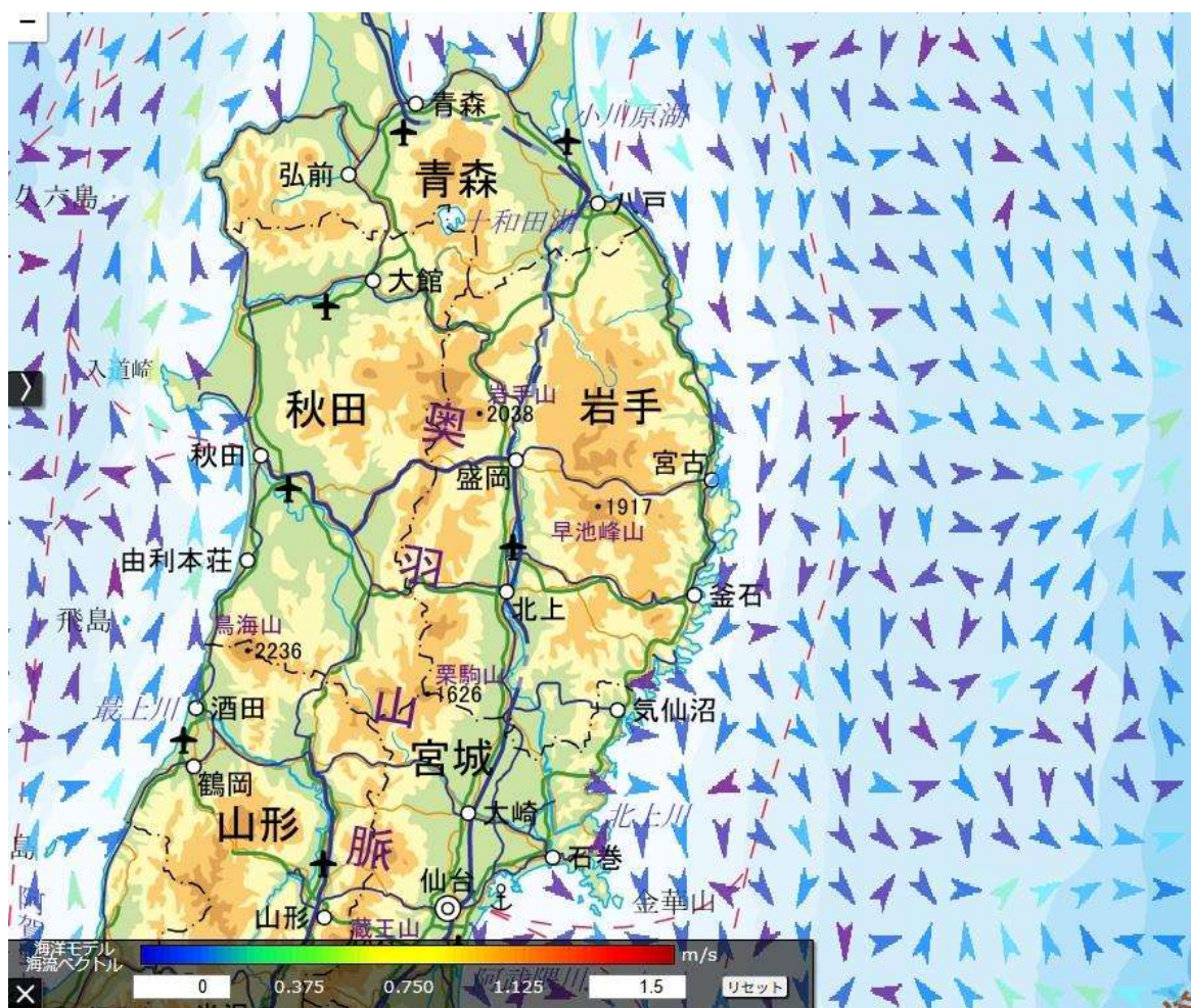
令和7年5月12日9時00分の潮流図（表面の解析値） 提供：宇宙航空研究開発機構・海洋研究開発機構（JAXA）
