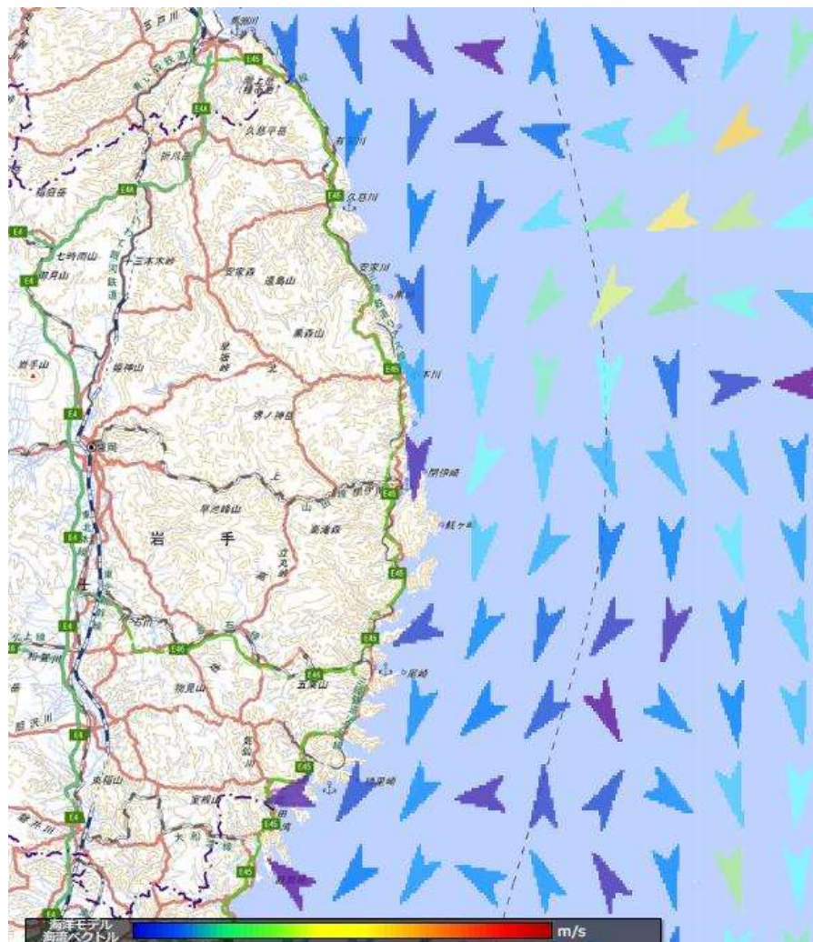
図1. 令和7年10月2日13時00分 本県沿岸潮流予想図（表面の解析値）
